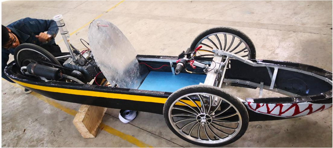
图 9 Honda 三代车
